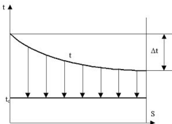
Fig. 4 Răcirea agentului de lucru în timpul cedării de căldură
