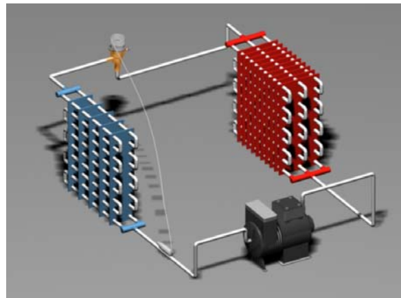
Fig. 9 Instalație frigorifică cu ventil de laminare termostatic
