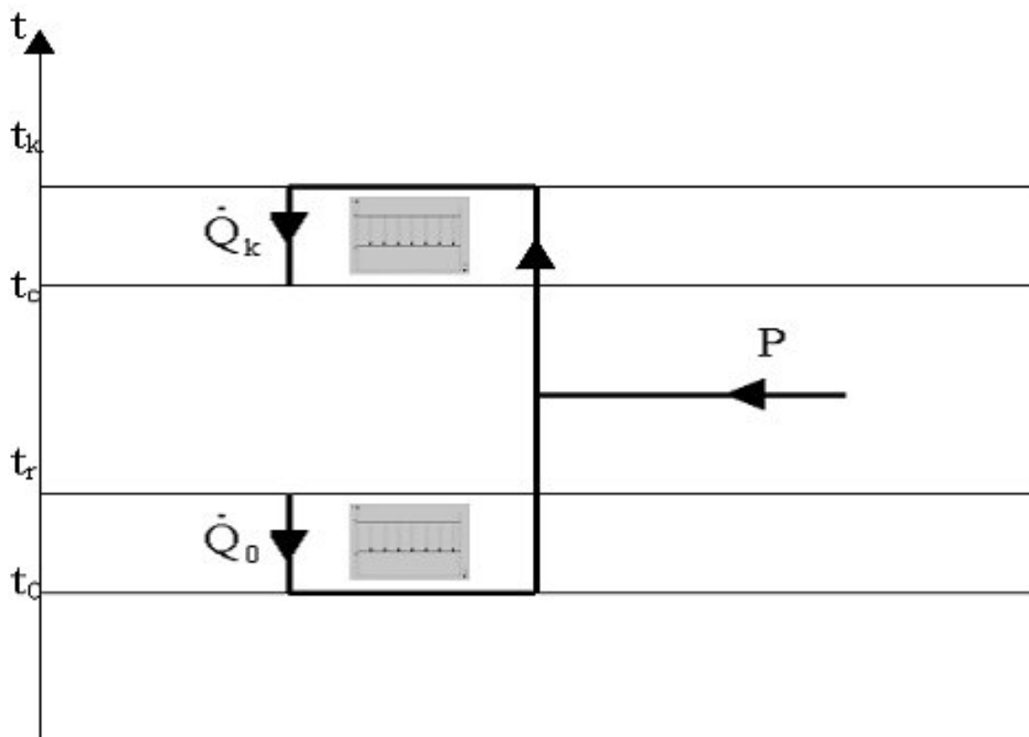
Fig. 6 Schema fluxurilor energetice din instalațiile frigorifice și pompele de căldură
