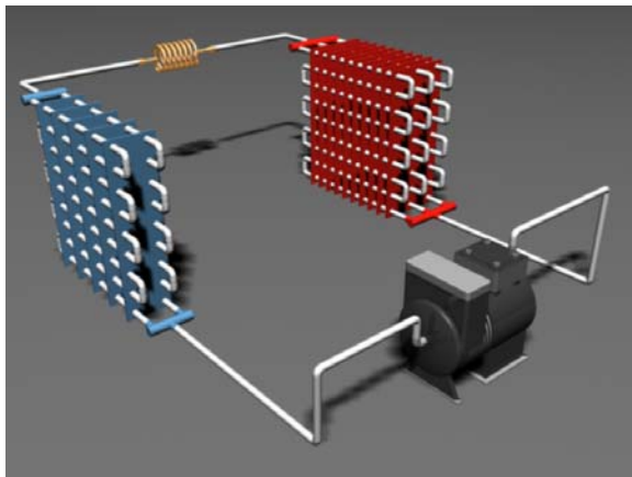
Fig. 8 Instalație frigorifică cu tub capilar
