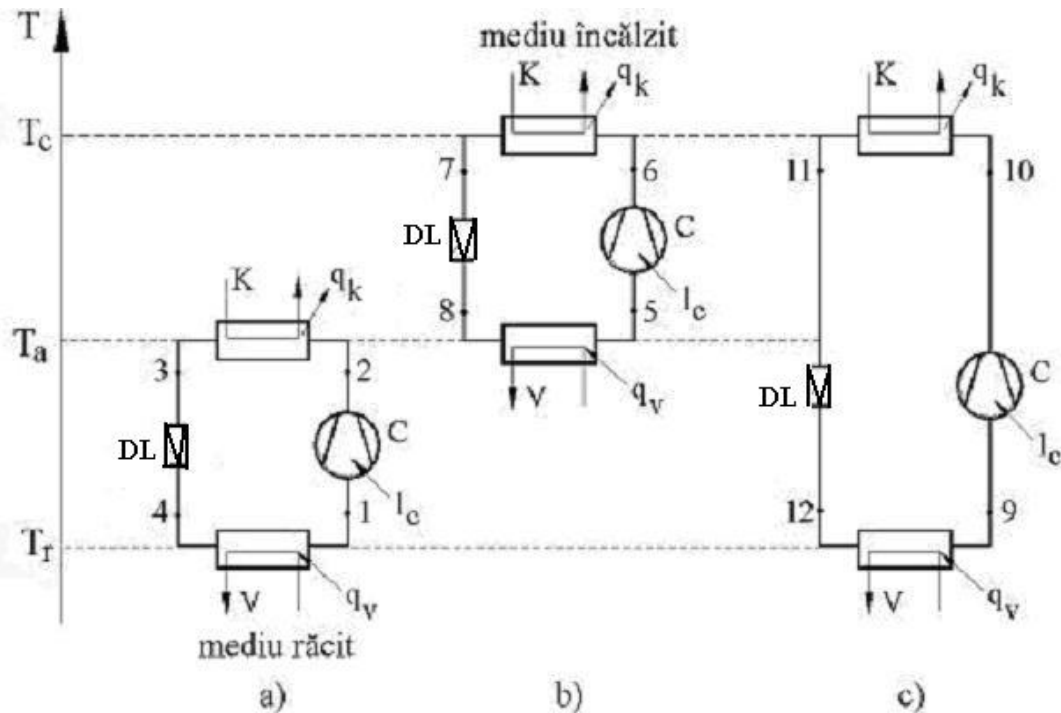
Fig. 10 Scheme de instalații funcționând după cicluri termodinamice inversate a) Instalație frigorifică; b) Pompă de căldură; c) Instalație combinată.
