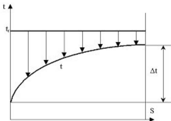
Fig. 2 Încălzirea agentului de lucru în timpul preluării de căldură
