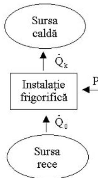
Fig. 1 Schema energetică a instalațiilor frigorifice și a pompelor de căldură
